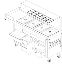
yemek dağıtım arabası mobile bain marie
